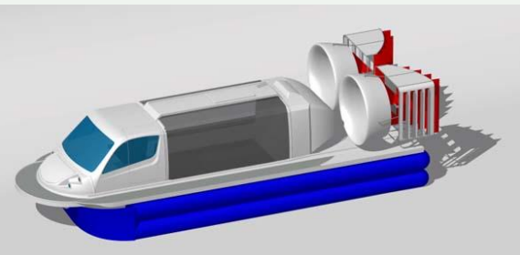
Versión: plataforma cubierta
